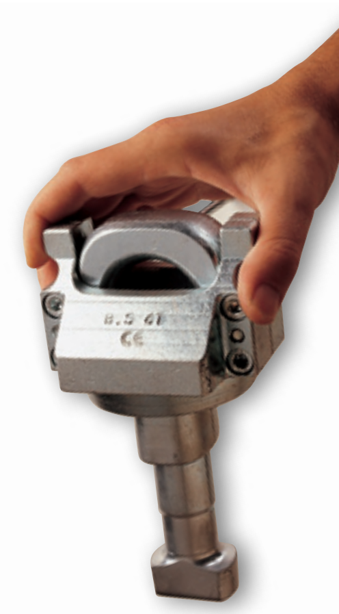
Cravatta per semplice e veloce staffatura a taglio Shear tie for simple and fast reinforcement
