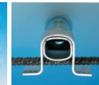
Cravatta per semplice e veloce staffatura a taglio Shear tie for simple and fast reinforcement
